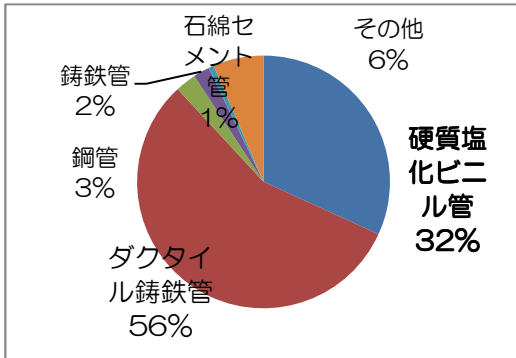
水道管種別管路延長((累積) (2016年度) 総延長(累積) 676,496km
